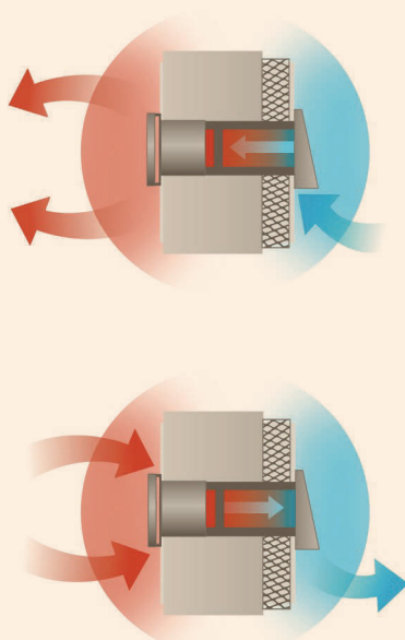
Zwei dezentrale Lüftungsgeräte mit alternierendem Betrieb mit Wärmerückgewinnung
